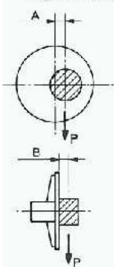
Diagrama de cargas
